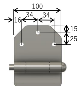
SPHC t=4.5 穴位置：全共通 ピン径：12.7mm
