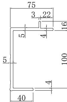
TSC (2.85kgf/m)
