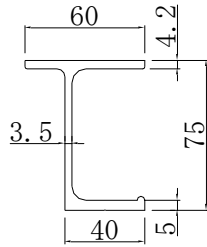
TYD (1.92kgf/m)
