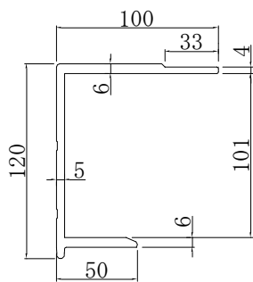
TSU (3.65kgf/m)
