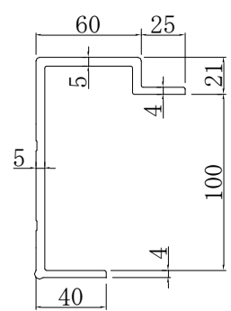
TSE (3.32kgf/m)
