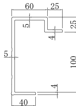
TSB (3.43kgf/m)
