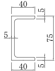
TYG (1.98kgf/m)
