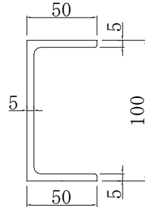
TYE (2.59kgf/m)
