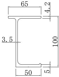
TYC (2.35kgf/m)
