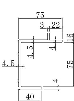
TSD (2.36kgf/m)
