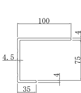
TSP (2.36kgf/m)
