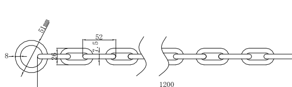
リング付チェーン
