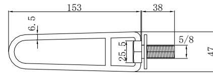
5/8x38 中柱締付ハンドル
