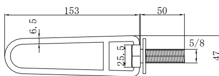
5/8x50 中柱締付ハンドル
