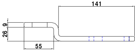
掛金9x65 3穴 26mm段
