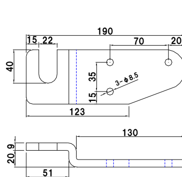
掛金 20mm段
