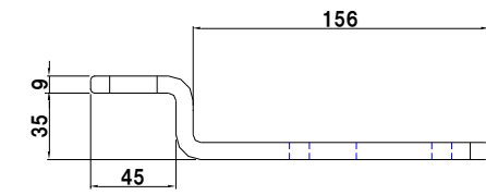
掛金9x65 3穴 35mm段
