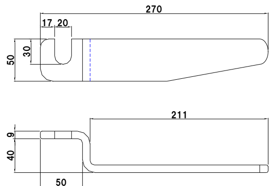
掛金9x50 40mm段
