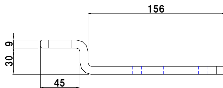
掛金9x65 3穴 30mm段
