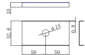
根太座金
