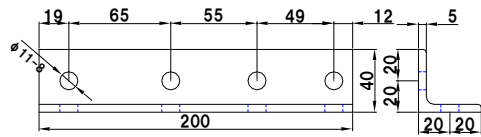
アングルピース L
