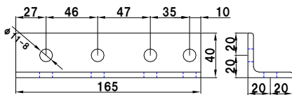
アングルピース S
