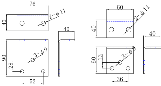
クロスメンバークリップ VC
