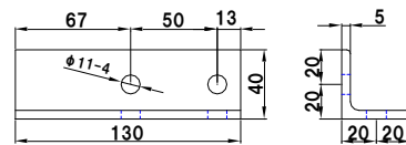
アングルピース MB
