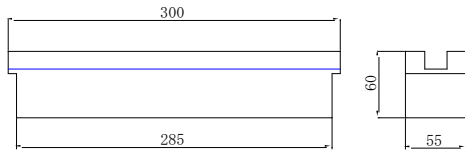
デスタンスピース285
