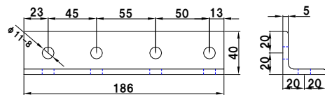
アングルピース MA
