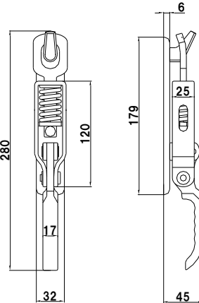
エビ金 鍛造 270 6t座付
