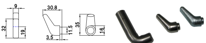
エビ金 鍛造フック受
