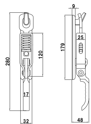
SUSエビ金鍛造270 9t座付
